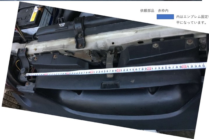
幅寸法 (W)
